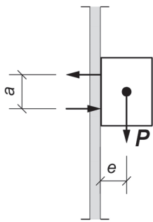
Abb. 108: Bei der Konsollast P darf die Exzentrizität e , d. h. der Abstand der vertikalen Wirkungslinie von der Wandoberfläche, nicht größer als 300 mm sein. Der Hebelarm a der entstehenden Horizontalkräfte muss mindestens 300 mm betragen.
