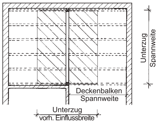
Abb. 92: Grundriss Balkenlage
