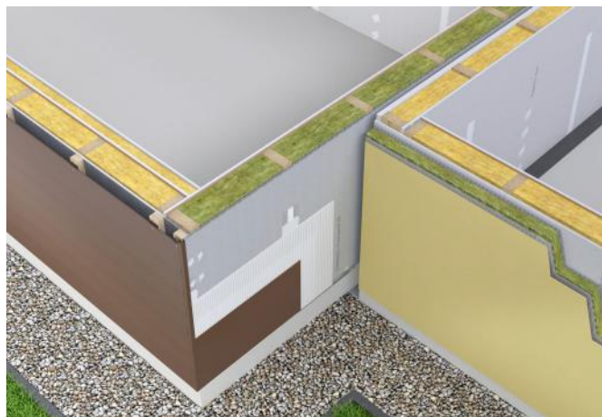
Abb. 25: Gebäudeabschlusswände (F 30-B/F 90-B) mit Prüfzeugnis. Bild: James Hardie Europe.
